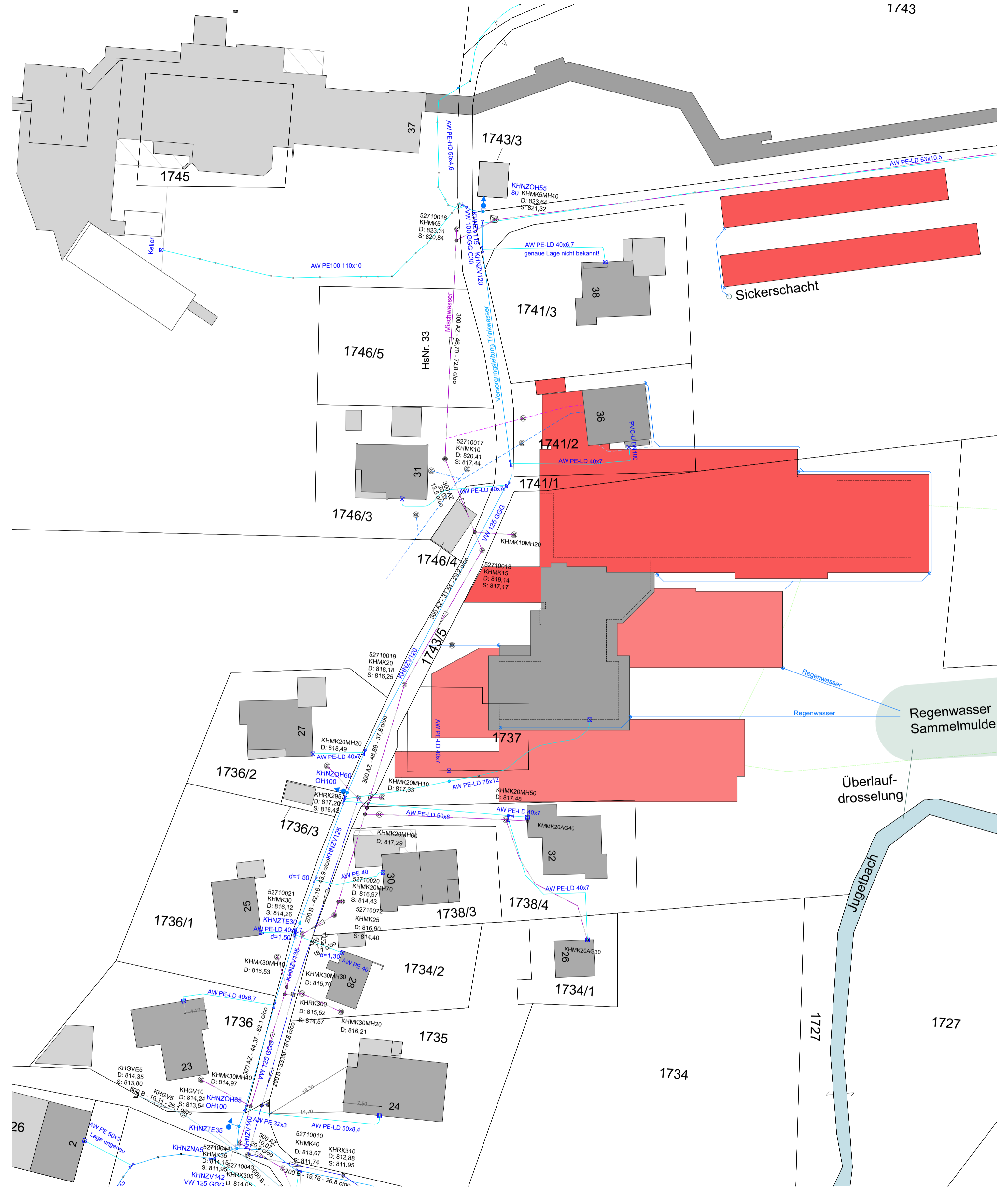
geplante Bebauung mit unveränderten Brauch- und Schmutzwasseranschlüssen
