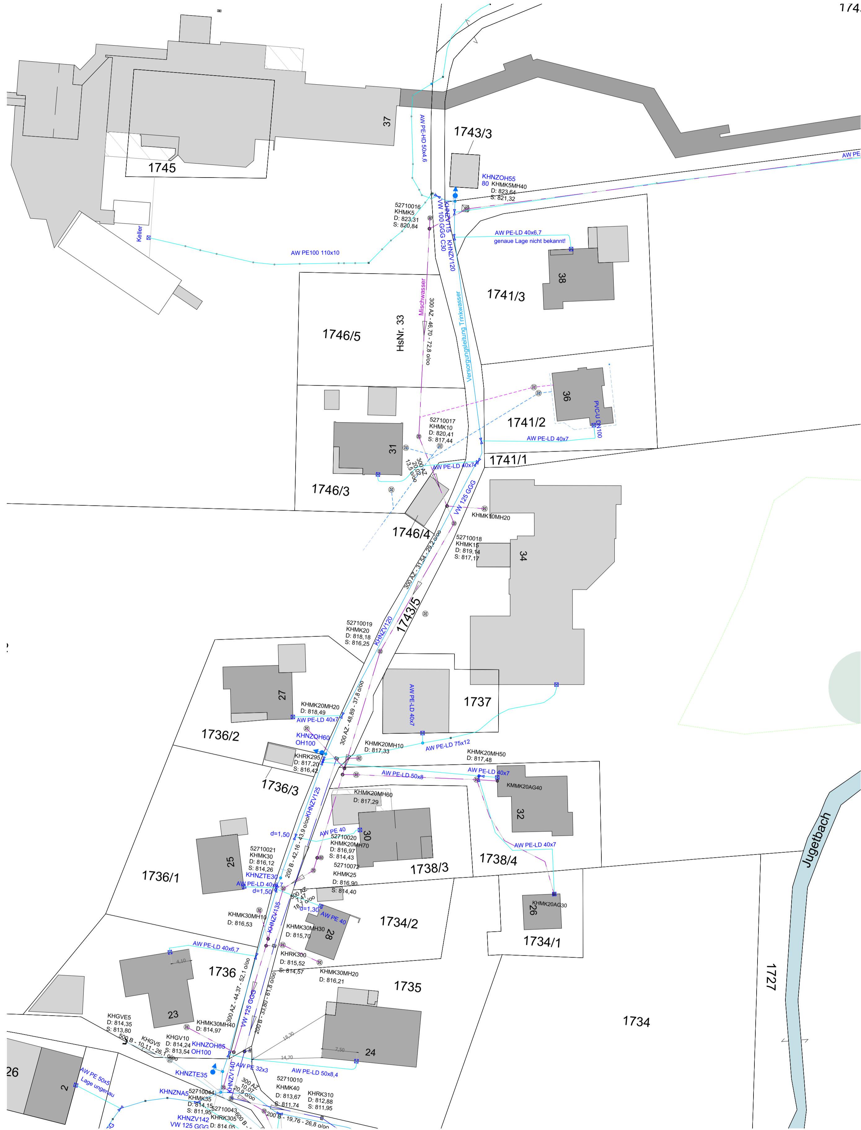
Ist-Zustand Bebauung mit Brauch- und Schmutzwasseranschlüssen
